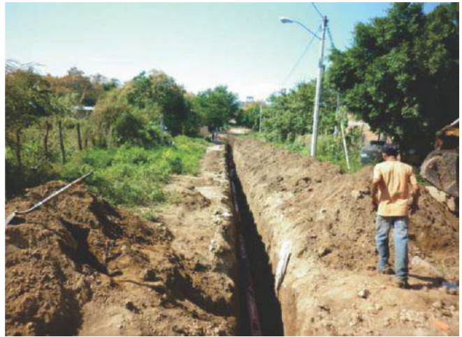
DRENAJE DE LA COMUNIDAD DE EL TERRERO Y LÍNEA DE CONDUCCIÓN DEL AGUA POTABLE DE LA COMUNIDAD DE SAN FRANCISCO
